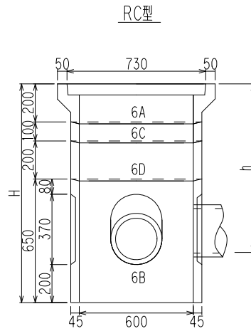
雨水樹 RC型
