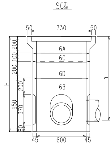
汚水樹 SC型
