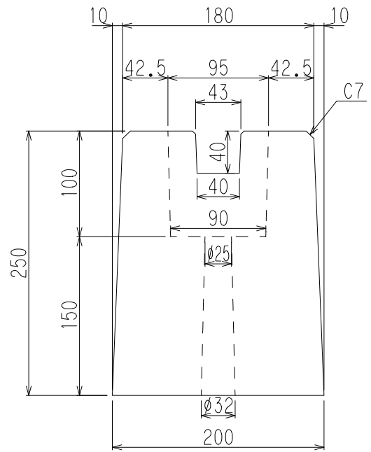
沓石2×4フ'ロック90用 参考重量 24kg
