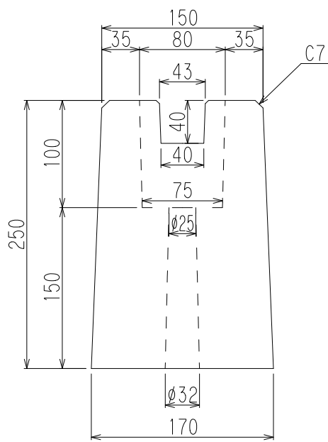
沓石2×4フ'ロック75用 参考重量 17kg
